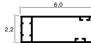
GA6 Guía Abierta de 6 x 2,2 cm
