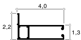
C4L Guía Cerrada de 4 x 2,2 cm Fijación Lateral
