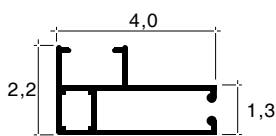
C4F Guía Cerrada de 4 x 2,2 cm Fijación Frontal
