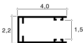
GA4 Guía Abierta de 4 x 2,2 cm
