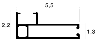
C5F Guía Cerrada de 5,5 x 2,2 cm Fijación Frontal
