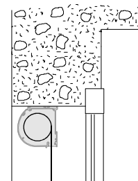
E-I Instalación Exterior Enrollamiento Interior
