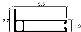
C5L Guía Cerrada de 5,5 x 2,2 cm Fijación Lateral
