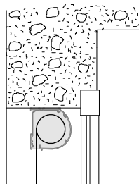
E-E Instalación Exterior Enrollamiento Exterior
