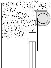
I-E Instalación Interior Enrollamiento Exterior
